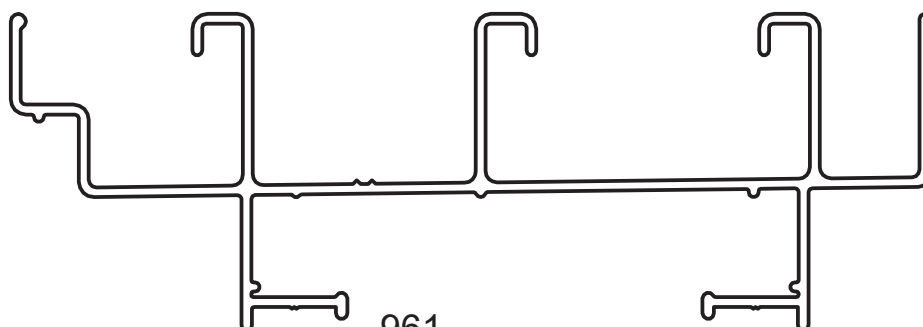
961 Marco de 3 guias Natural: 1,210 grs / mt Pintado: 1,269 grs / mt Paquetes de 4 barras Largo Barras 6.050mm
