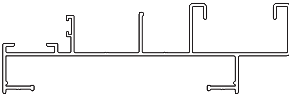
965 Marco de combinado Natural: 1,185 grs / mt Pintado: 1,242 grs / mt Paquetes de 4 barras Largo Barras 6.050mm
